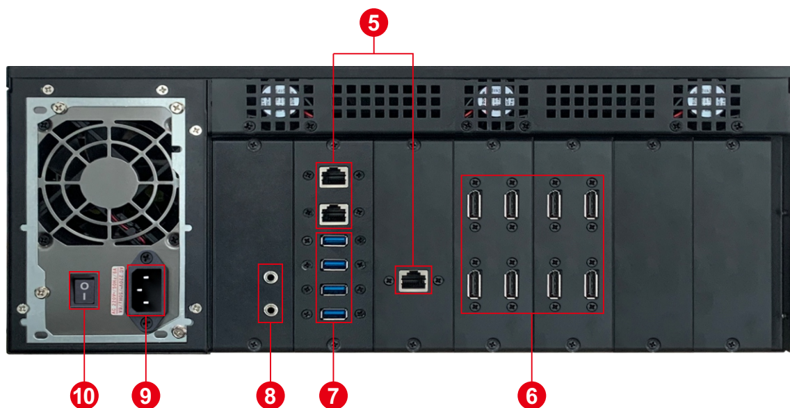
▲ 设备背面
